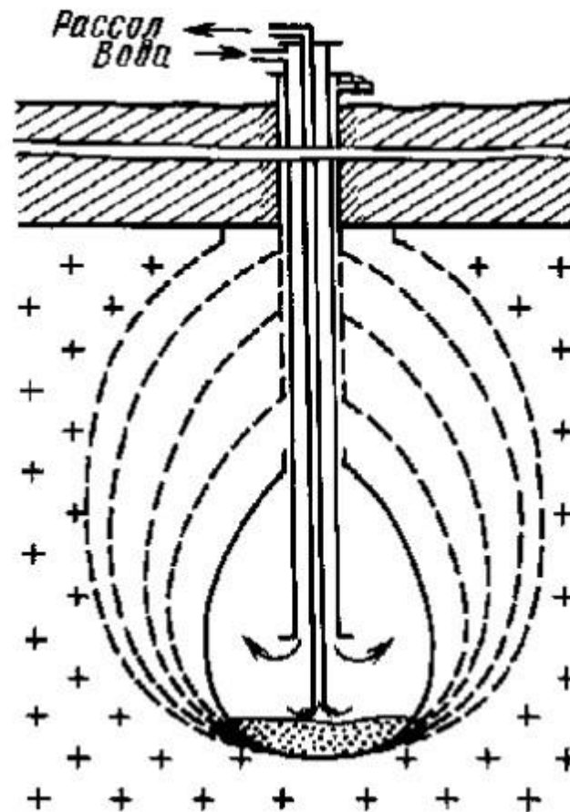
Рис.3. Схема разработки с использованием метода "без нерастворения"
