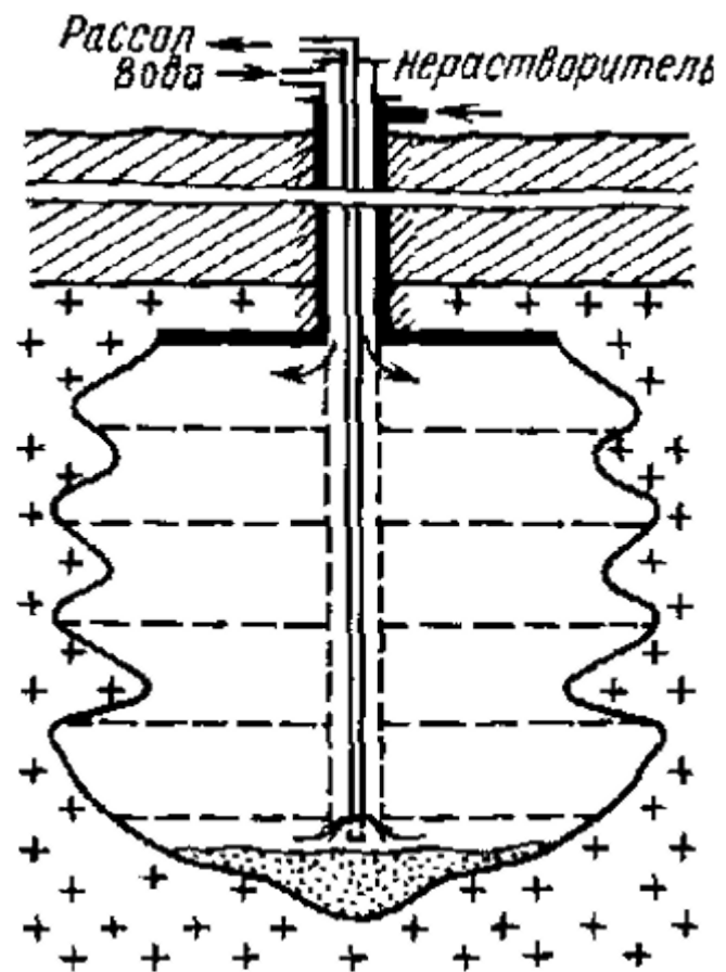
Рис.1. Схема разработки с использованием "послойного" (ступенчатого) метода
