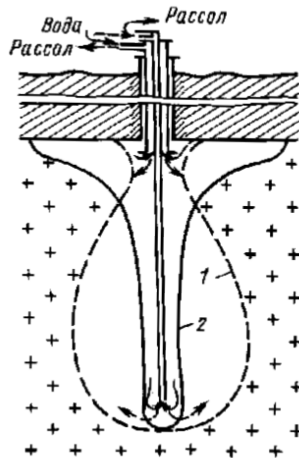
Рис.4. Схема разработки с использованием методов: 1 - прямотока; 2 - противотока
