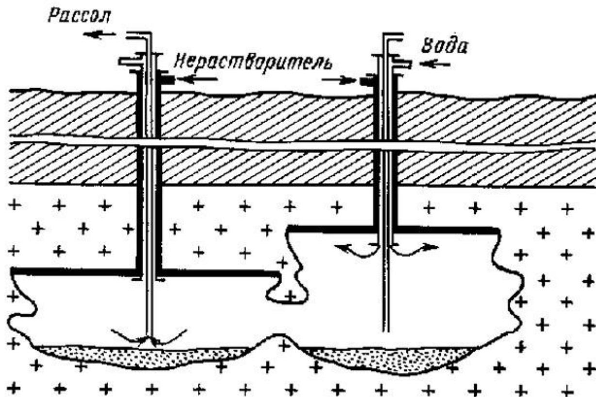
Рис.5. Схема разработки "батарейным" методом (сдвоенная камера)
