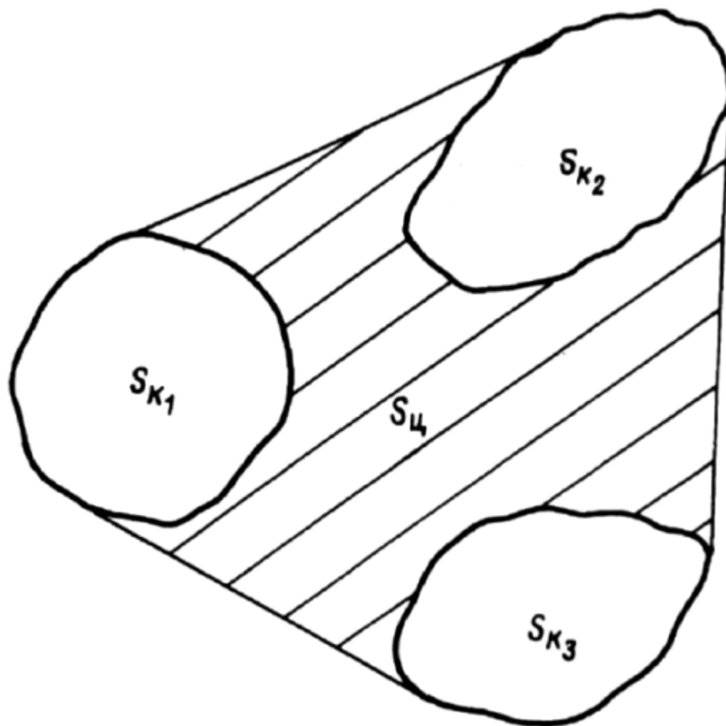
Рис.12. Схема к определению расчетного коэффициента извлечения междукammerного целика Категория устойчивости междукammerного целика определяется в зависимости от степени нагруженности \bar{C} :
