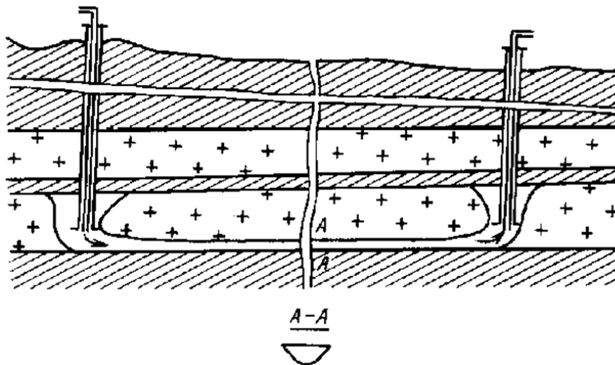
Рис.7. Схема разработки сплошным растворением при сбойке скважин гидроразрывом с последующим размывом канала сбойки
