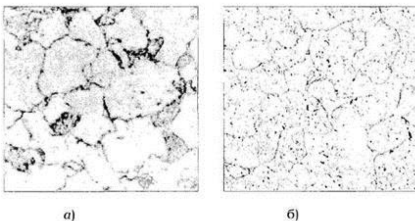
Рисунок 8 - Микроструктура сталей 12X1MΦ (а) и 15X1M1Φ (б).
