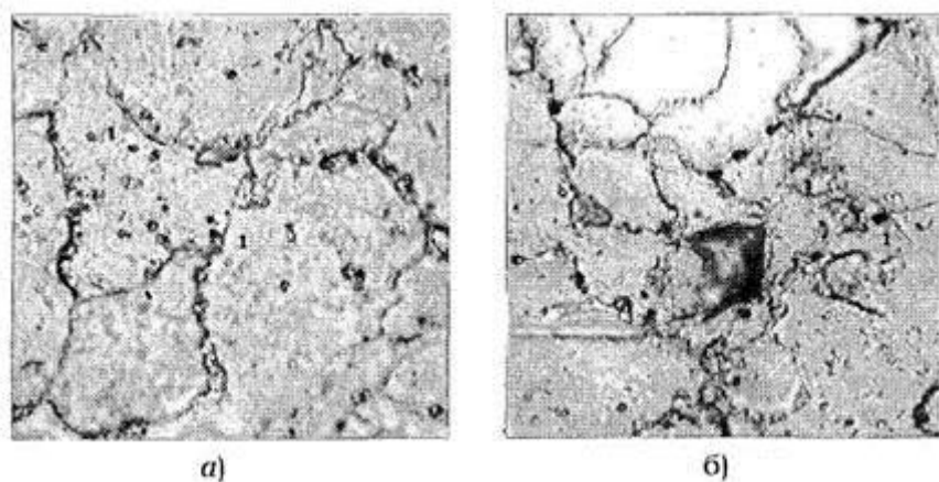
Рисунок 13 - Микроструктура стали 12Х1МФ
