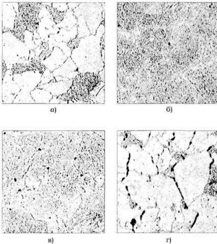
Рисунок 4 - Микроструктура сталей 12X1MФ (а, г) и 15X1M1Ф (б, в)
