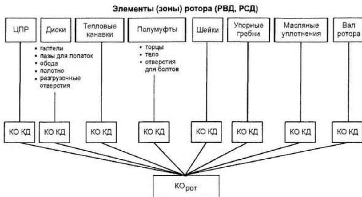
Рисунок 3 - Блок-схема экспертизы состояния ротора
