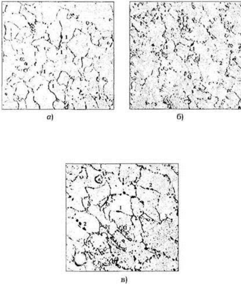
Рисунок 14 - Микроструктура стали 12Х1МФ
