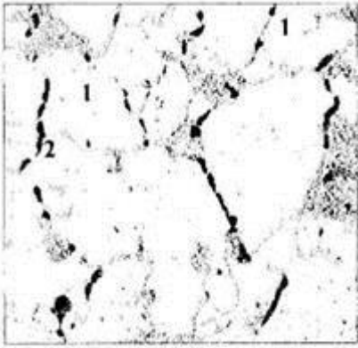
Рисунок 9 - Микроструктура стали 12Х1МФ. Микрошлиф (500-кратное увеличение) Границы зерен тонкие, четкие. Единичные микропоры (1), цепочки микропор (2)
