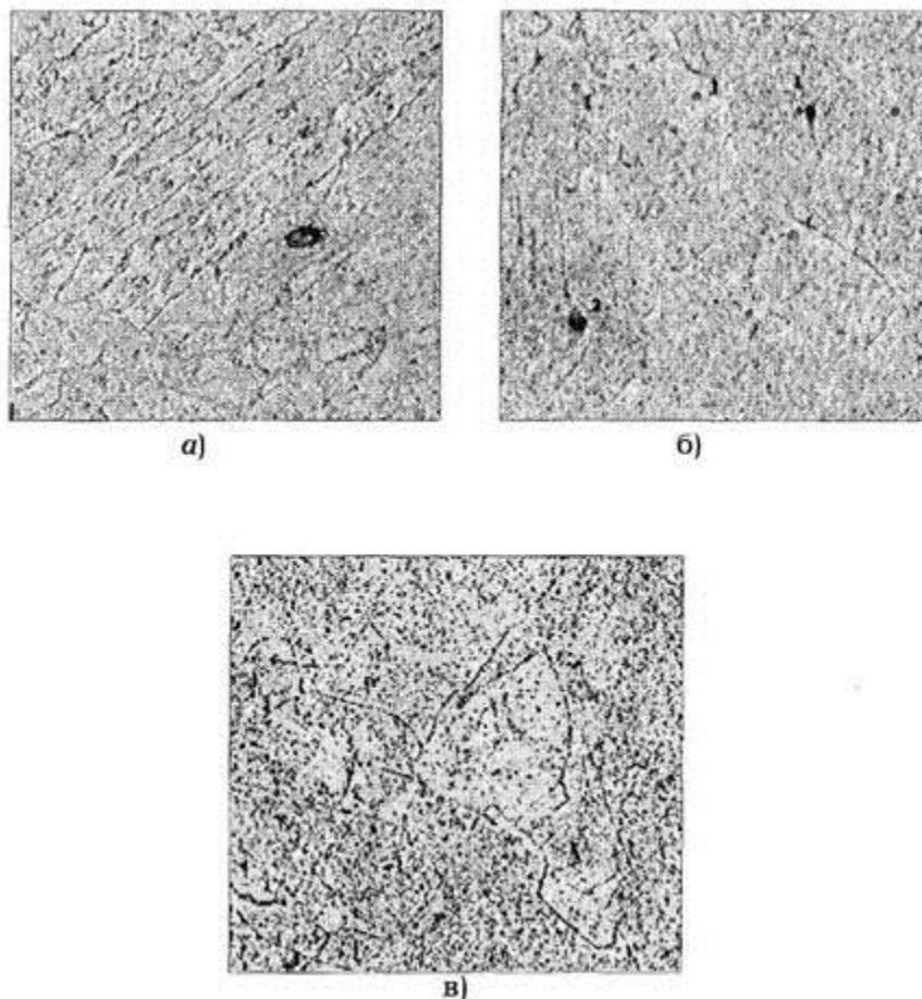
Рисунок 12 - Микроструктура стали 12Х1МФ Микрошлифы (500-кратное увеличение) а) единичное неметаллическое включение; б) единичные изолированные поры (1), неметаллические включения (2); в) микропоры и неметаллические включения отсутствуют
