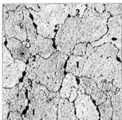
Рисунок 6 - Микроструктура стали 12Х1МФ. Микрошлиф (500-кратное увеличение). Микропоры округлой (1), каплевидной (2) и треугольной формы (3)
