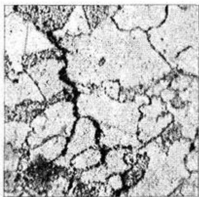
Рисунок 5 - Микроструктура стали 12Х1МФ. Микрошлиф (300-кратное увеличение). Зигзагообразные микротрещины по границам зерен
